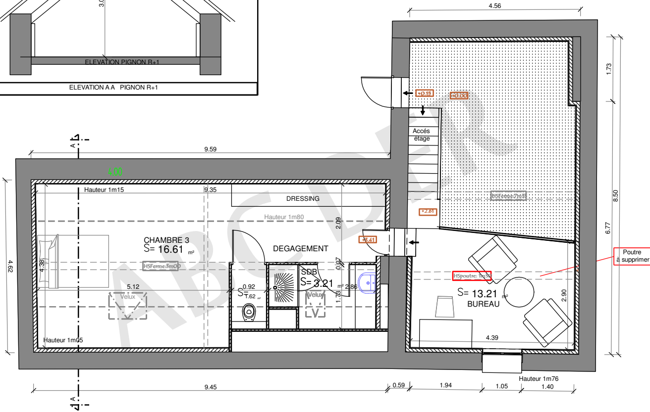
1 er Etage
